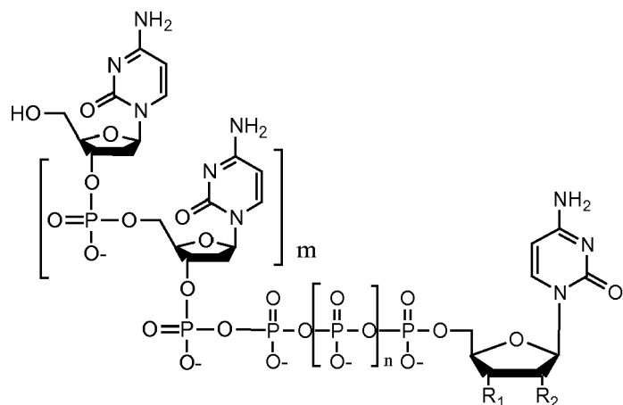
(dCp) m -(PO 4 ) n -dC
