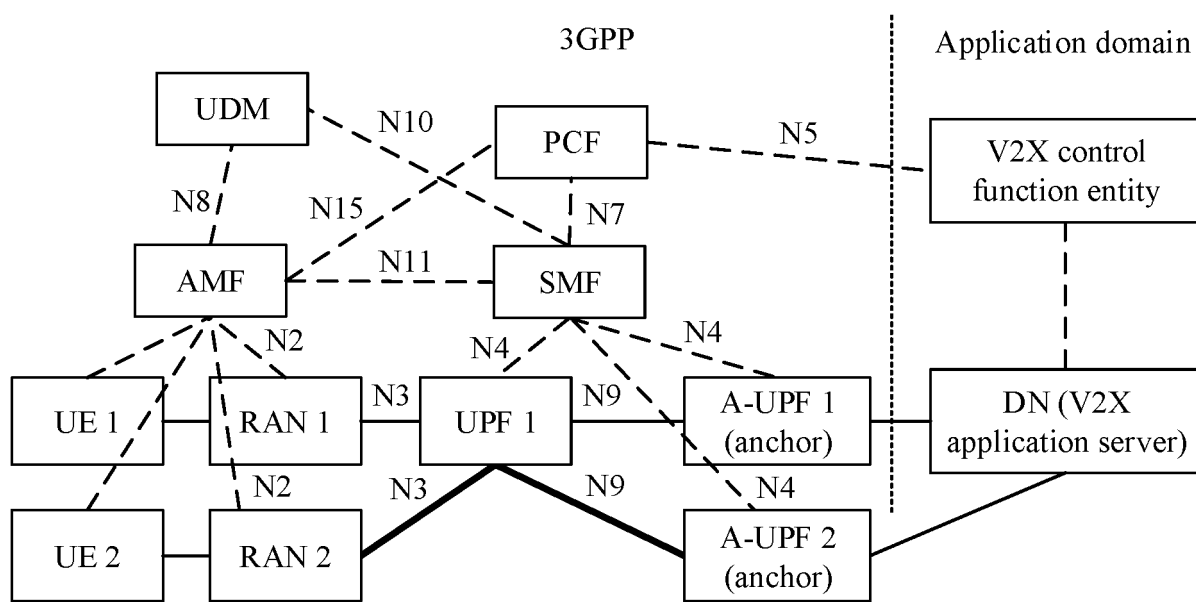
FIG. 10(b)
