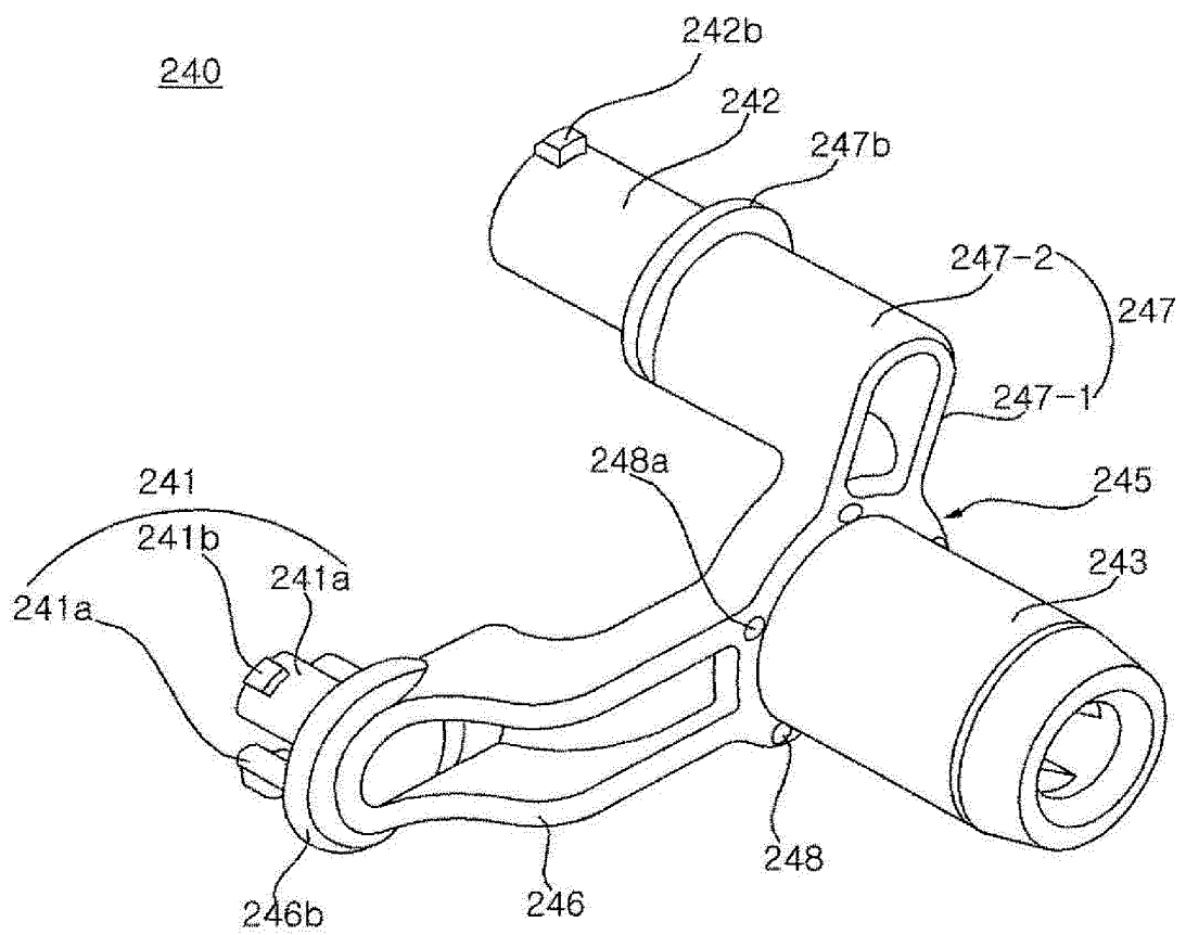
Fig. 26
