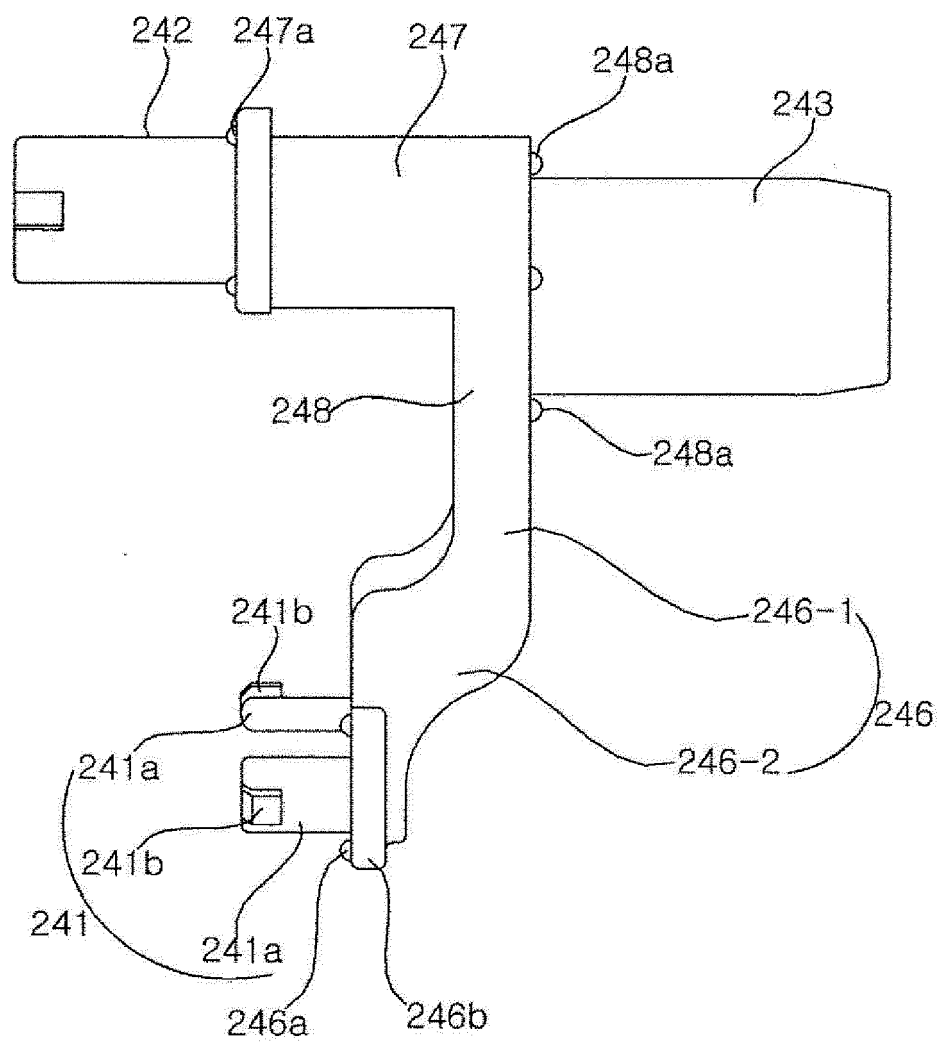
Fig. 27
