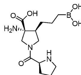
Serine AUC = 14784
