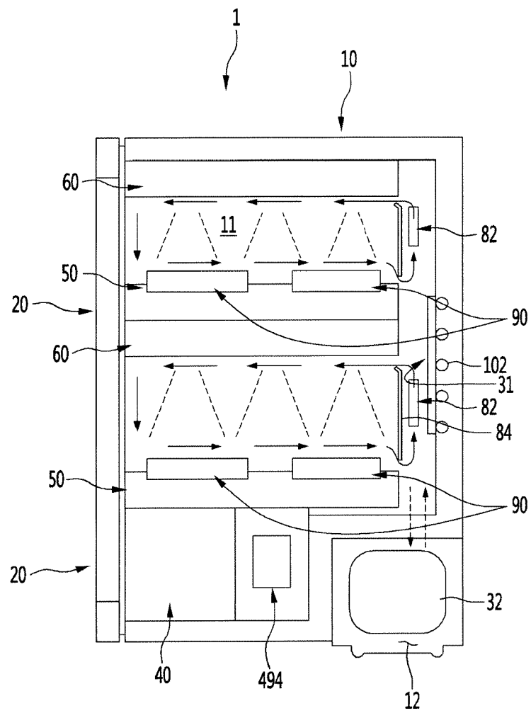
FIG. 48
