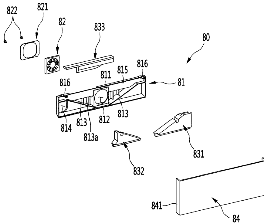
FIG. 36
