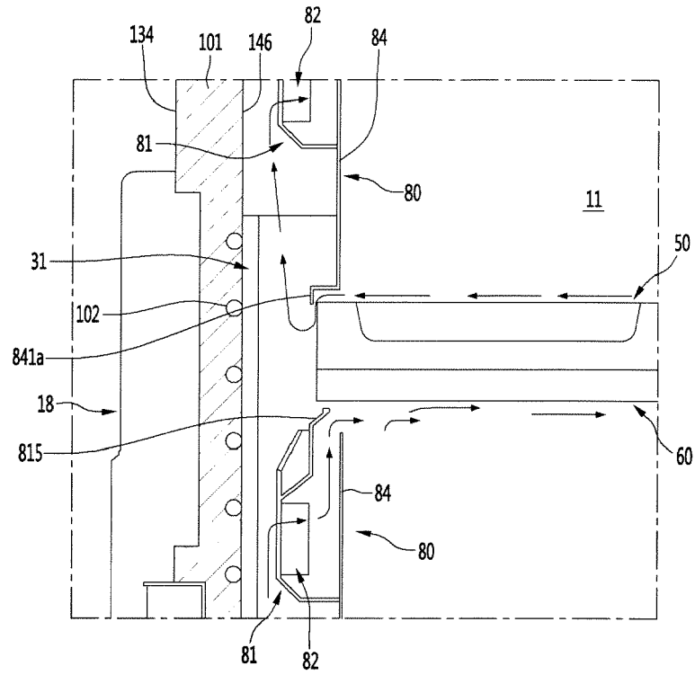
FIG. 41
