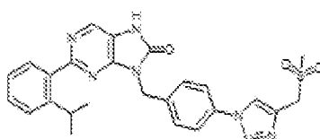
I-350. 2-(2-isopropylphenyl)-3-(4-((methylsulfonyl)methyl)-1H-1,2,3-triazol-1-yl)benzyl-7,8-dihydro-5H-purin-8-one
