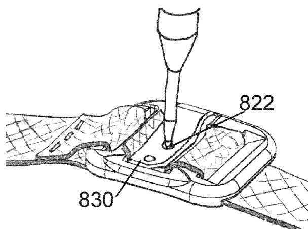
FIG. 76
