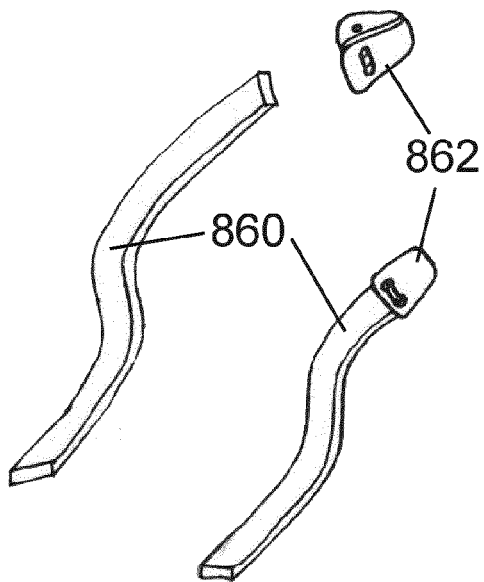
FIG. 79
