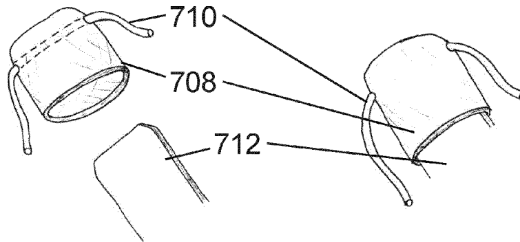
FIG. 67
