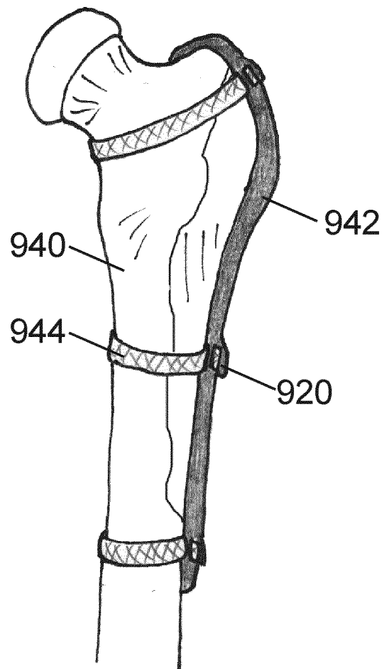
FIG. 88
