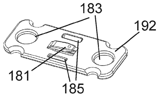
FIG. 12a
