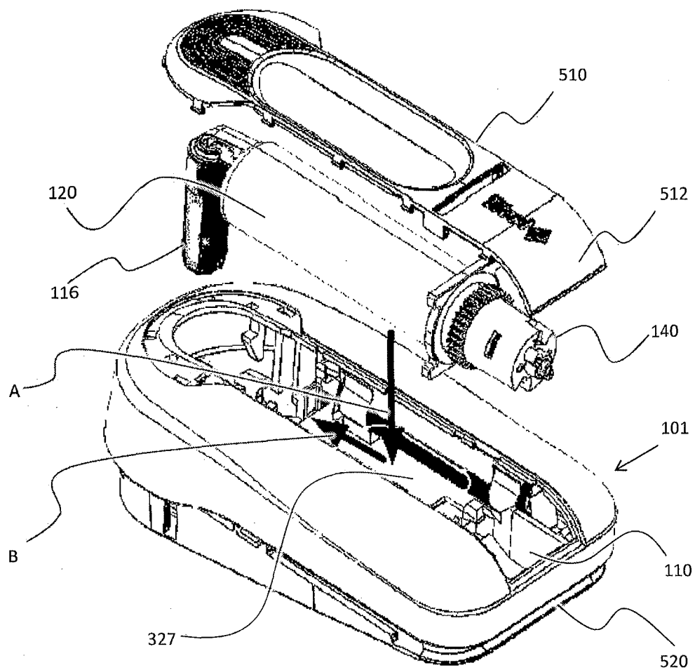
FIG. 5 Exemplary assembly
