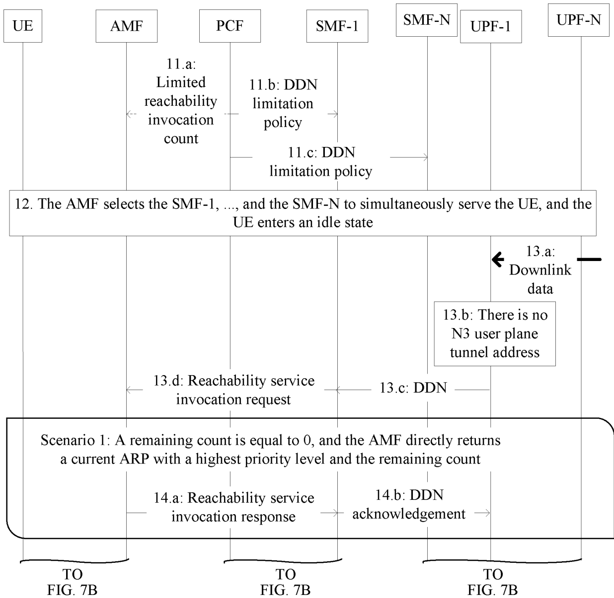
FIG. 7A
