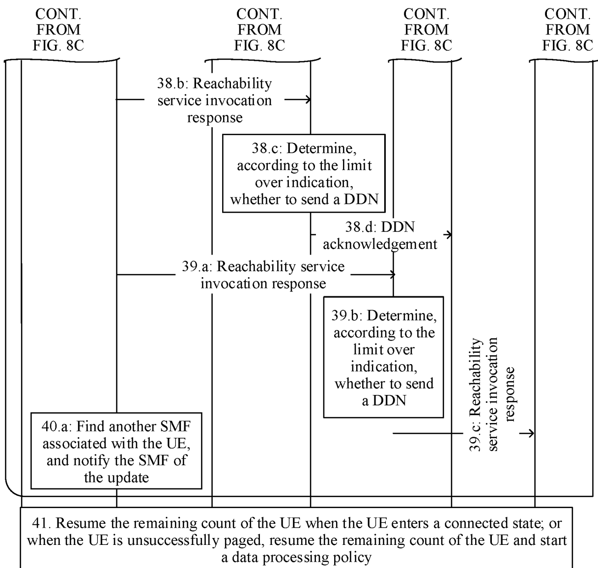
FIG. 8D
