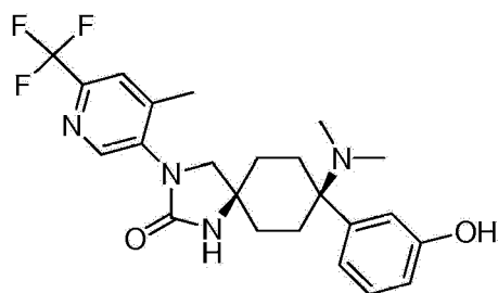
SC_3388
