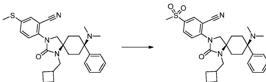
SC_3008
