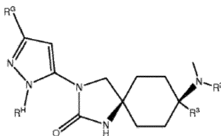
(XI)
