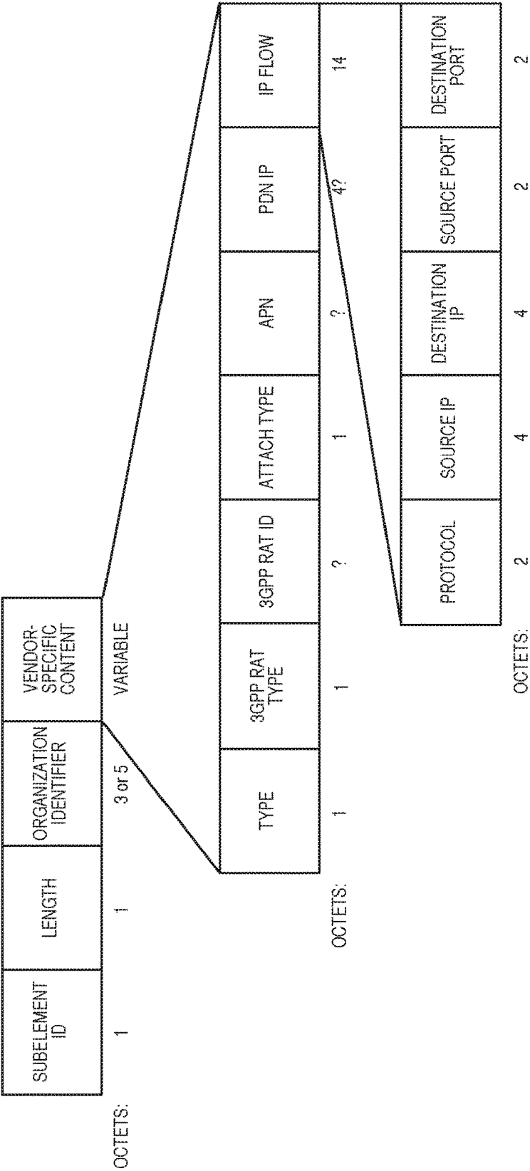
FIG. 6C
