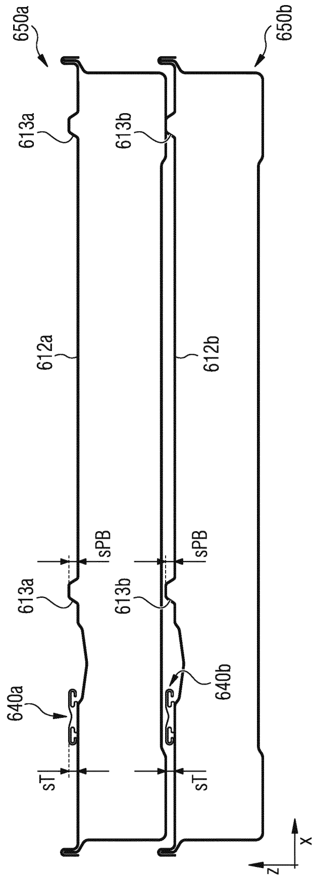
FIG. 6f E-E
