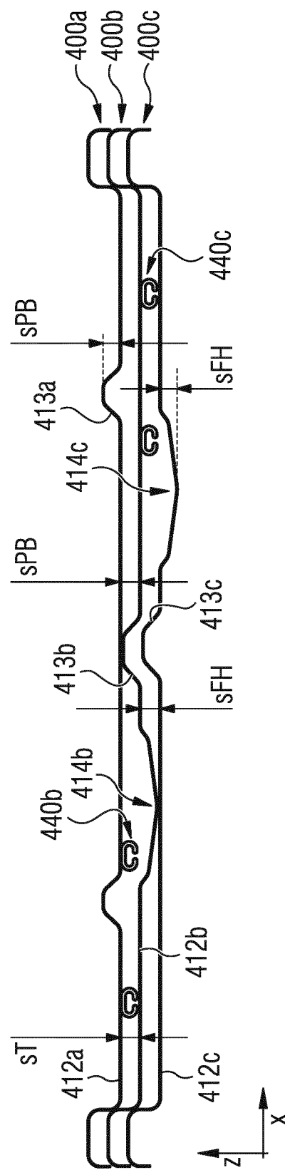
FIG. 4d C-C
