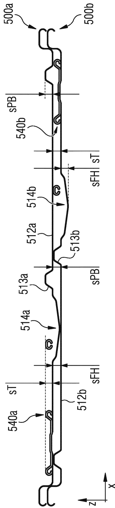
FIG. 5d D-D
