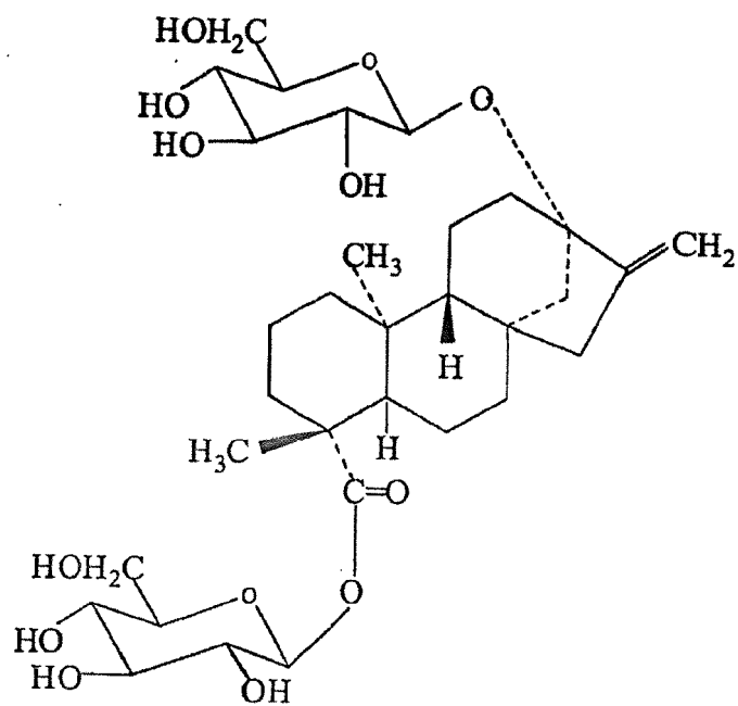
Rubusoside
