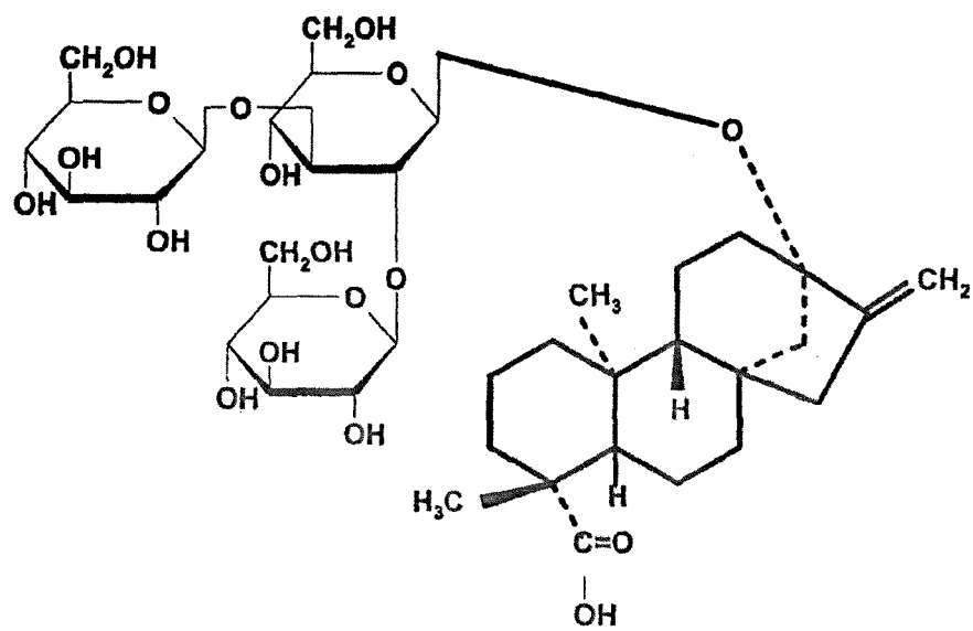
Rebaudioside B
