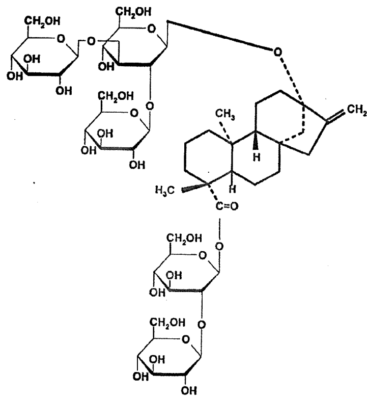
Rebaudioside D
