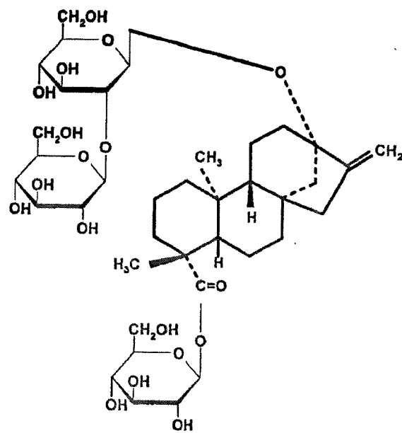
Stevioside
