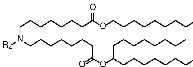
(IIa),
