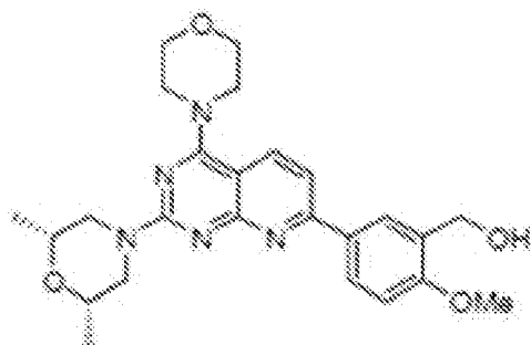
KU-0063794
