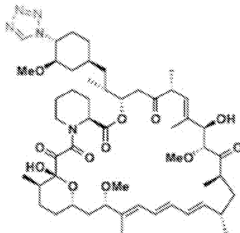
Zotarolimus (ABT-578)
