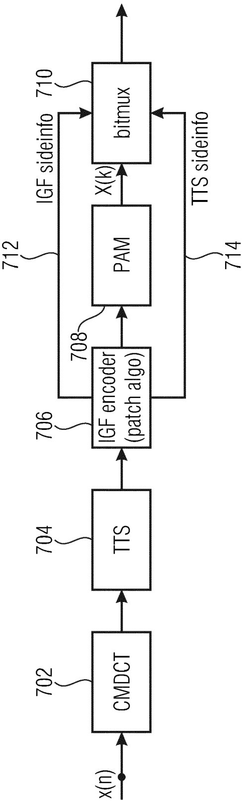
FIG 7A (ENCODER)
