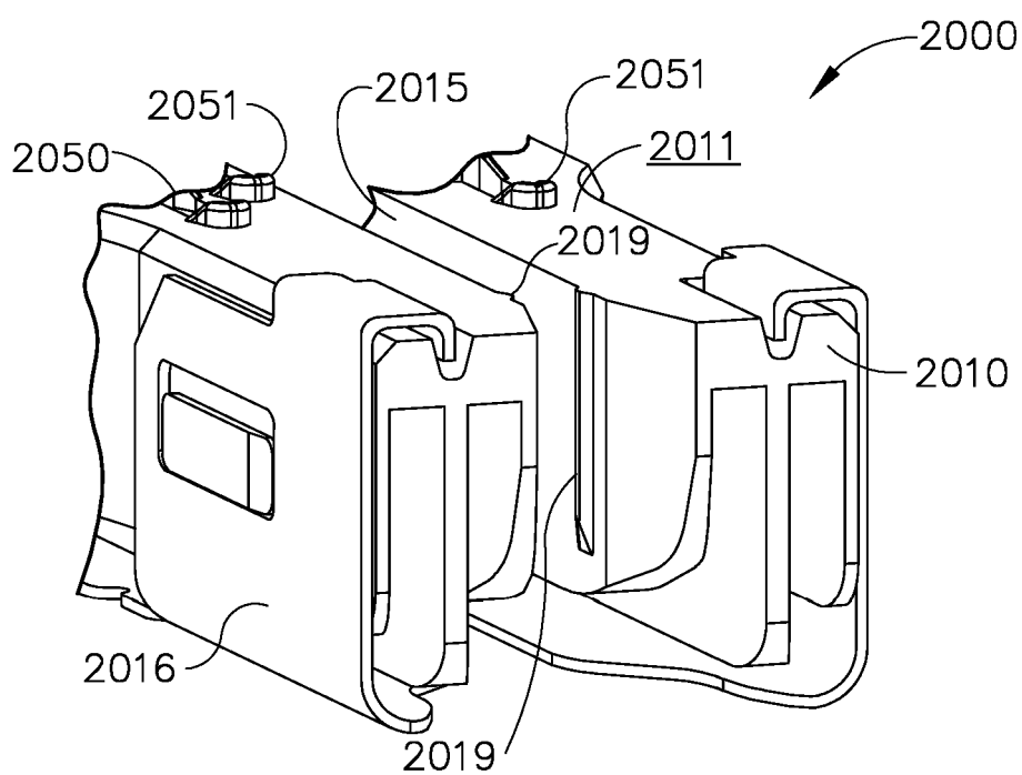
FIG. 54C
