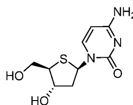
T-dCyd
