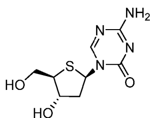
5-aza-T-dCyd
