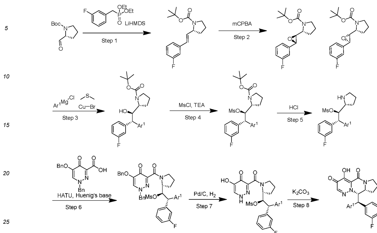
Scheme D.
