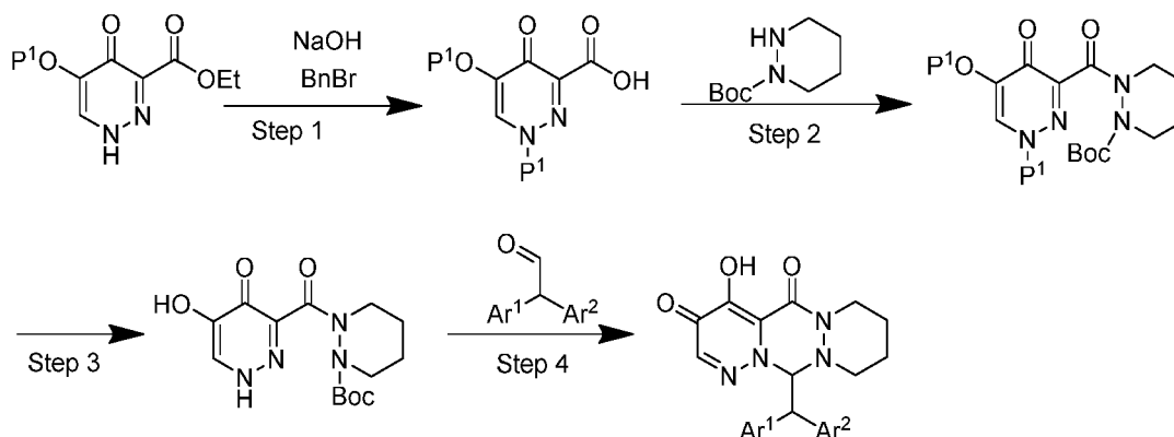
Scheme A.
