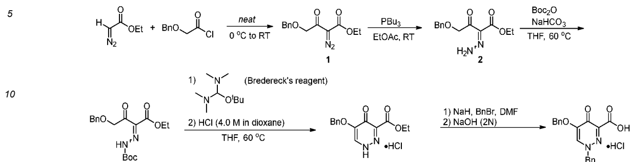
Scheme B.
