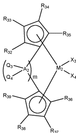
[Formule chimique 3]
