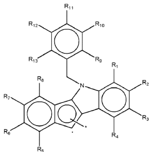
[Formule chimique 2b]
