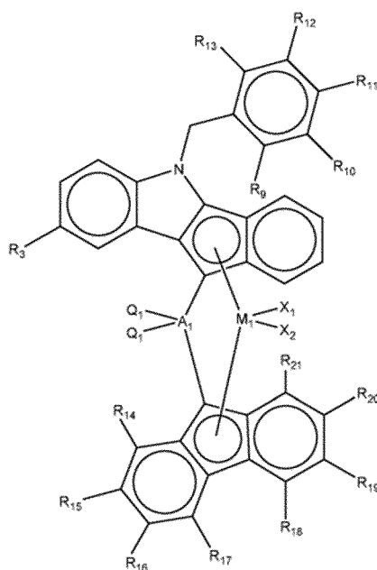
[Formule chimique 1-1]
