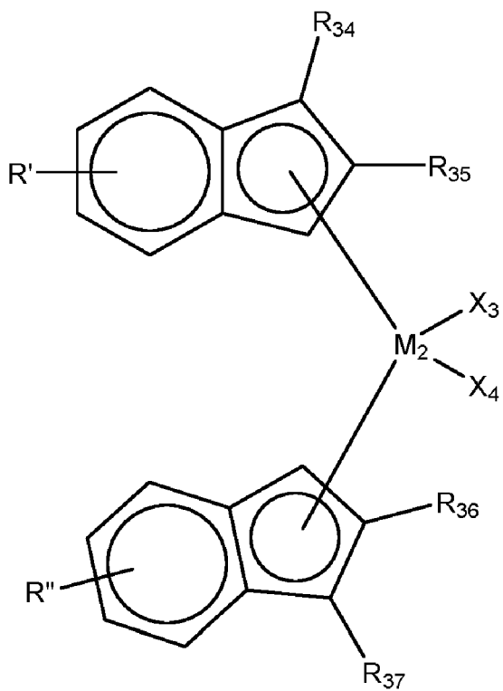
[Chemische Formel 3-3]
