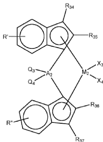
[Formule chimique 3-4]
