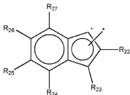
[Formule chimique 2e]
