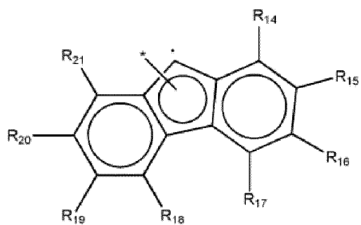
[Formule chimique 2c]
