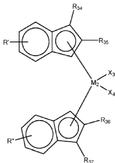
[Formule chimique 3-4]
