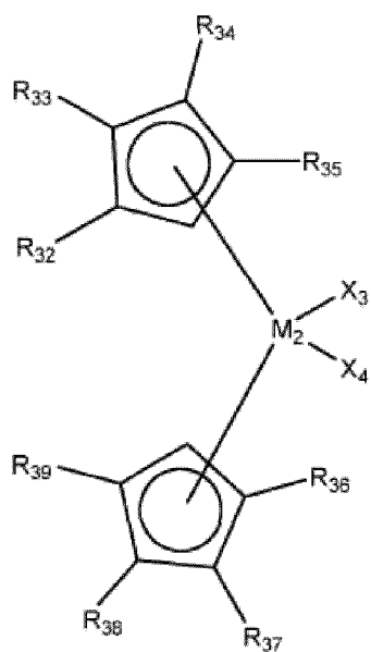
[Formule chimique 3-2]
