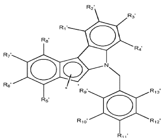
[Formule chimique 2c]
