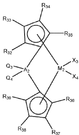
[Formule chimique 3-2]
