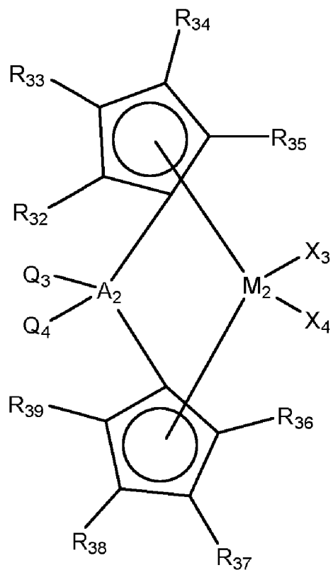
[Chemische Formel 3-3]
