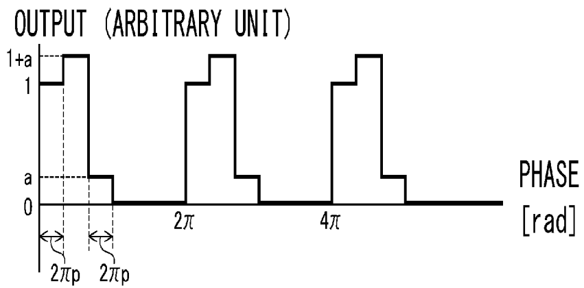
FIG.12C
