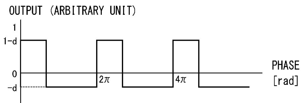
FIG.11B
