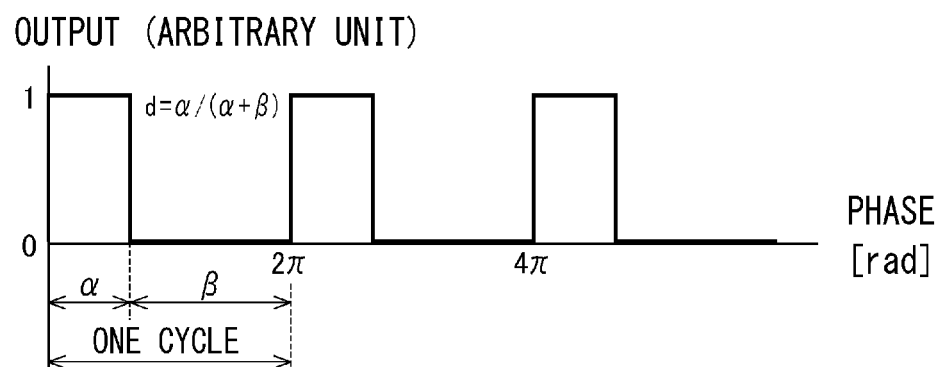
FIG.11A
