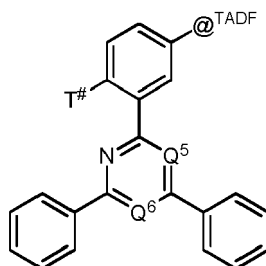
Formula LpT-I
