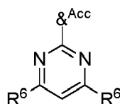
Formula A3
