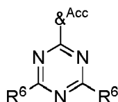
Formula A1
