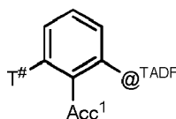
Formula TmL
