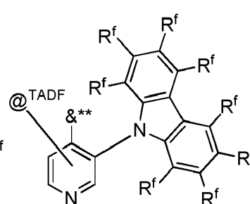
Formula B9*
