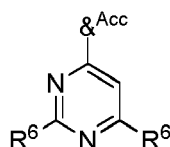
Formula A2
