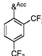
Formula A17
