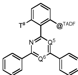
Formula TmL-I
