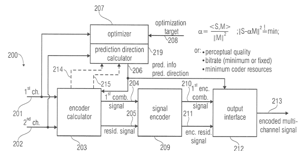
FIG 2 (AUDIO ENCODER)
