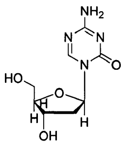
Decitabine
