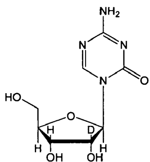
I-2
