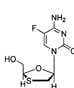
Emtriva
