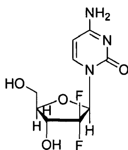
Gemcitabine
