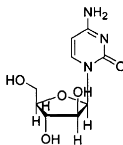
Cytarabine (Ara-C)
