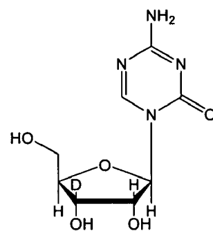
I-3
