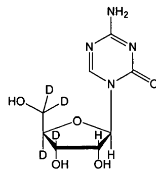
I-6
