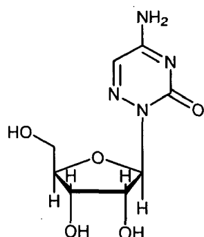
6-Azacytidine
