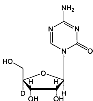
I-4
