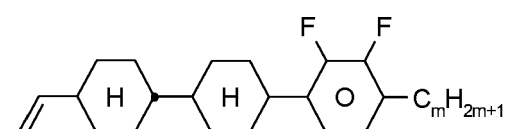
CCY-V-m
