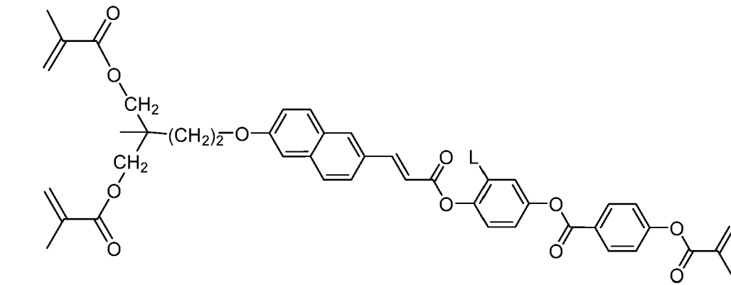
I-3-2a-5
