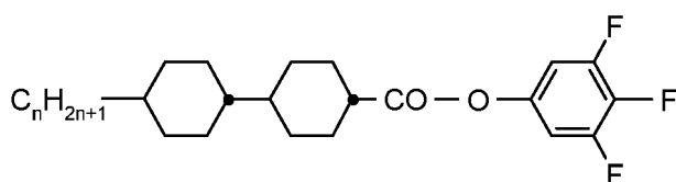
CCZU-n-F
