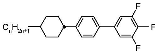
CPU-n-F
