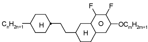
CETNap-n-Om
