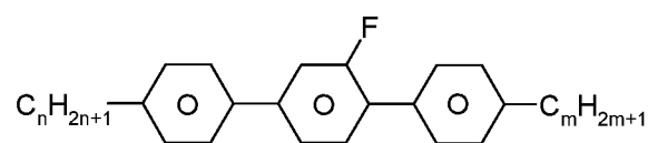
LY-n-(O)m
