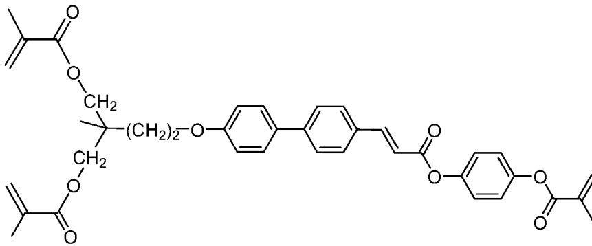
I-2-1a-10
