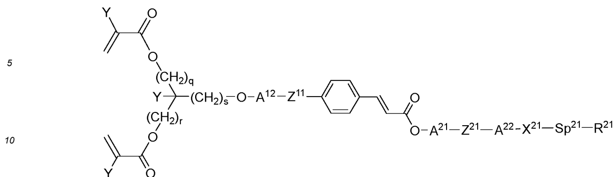
I-4-1
