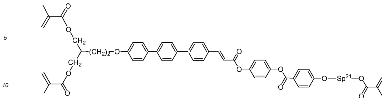
I-5-1a-1
