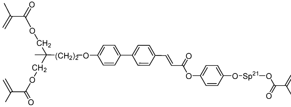
I-2-1a-9
