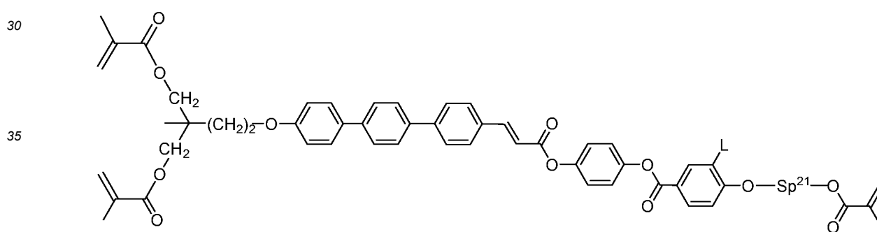
I-5-1a-27
