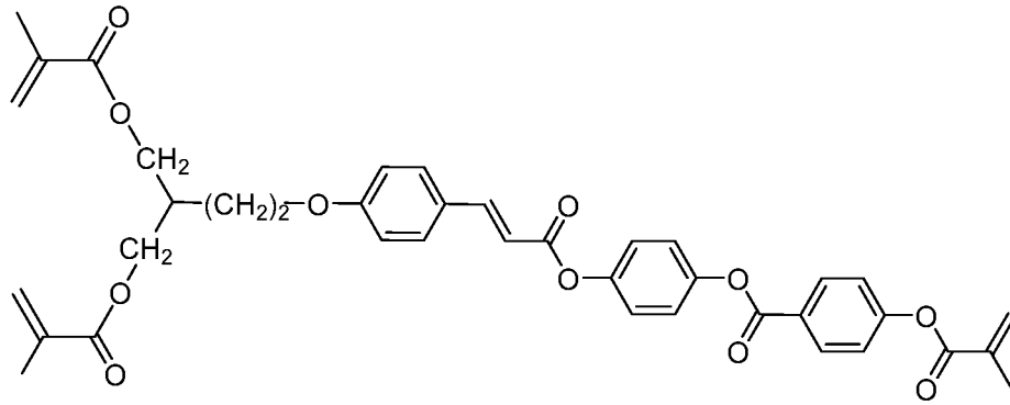
I-3-1a-3
