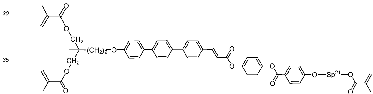
I-5-1a-15
