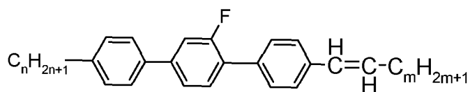
PGP-n-Vm
