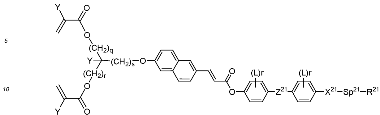
I-3-2a
