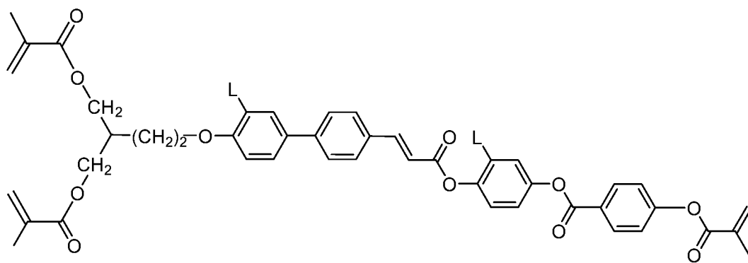
I-4-1a-6
