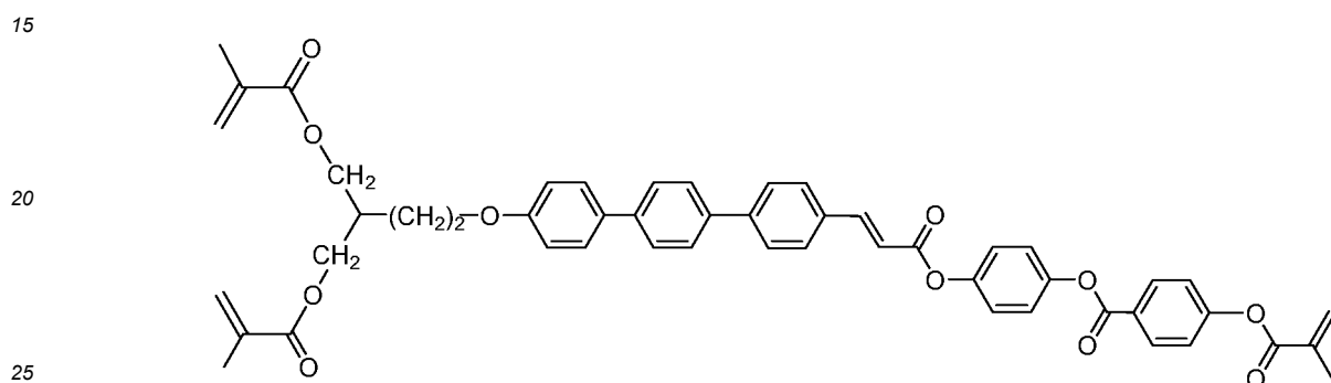
I-5-1a-2
