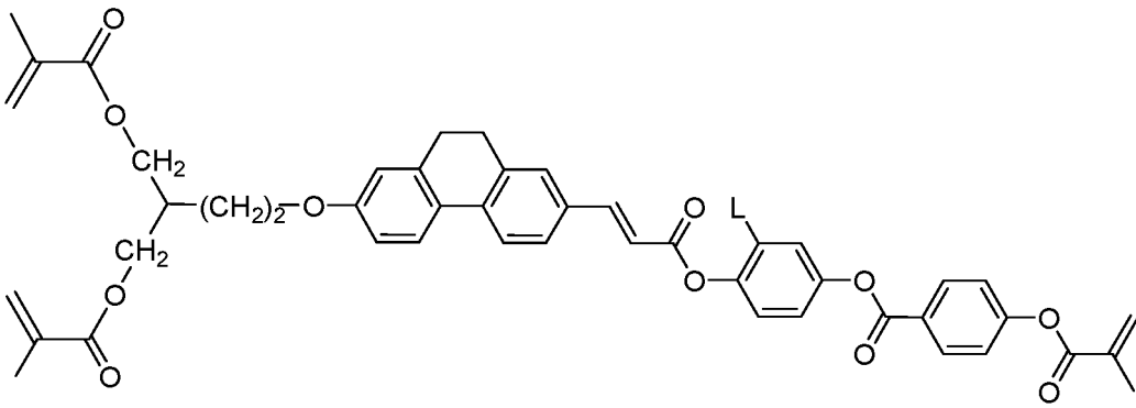
I-3-3a-2
