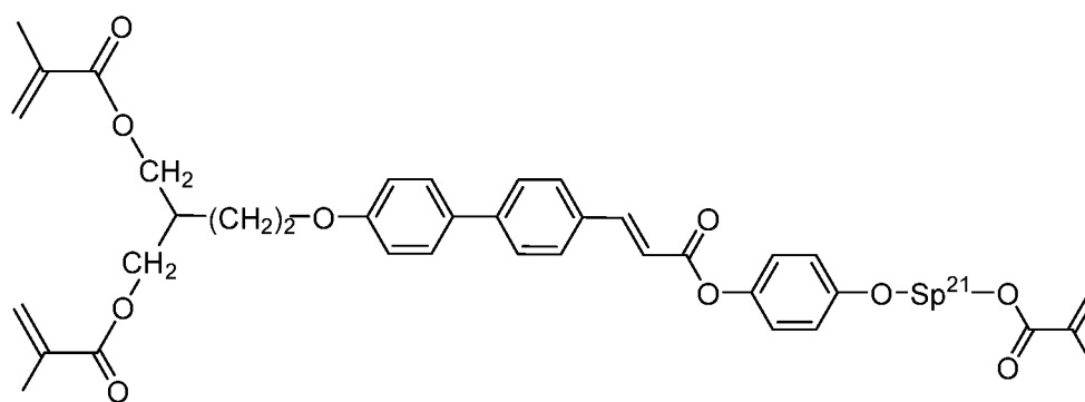
I-2-1a-1
