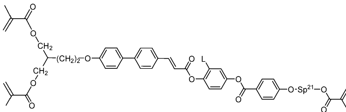
I-4-1a-7
