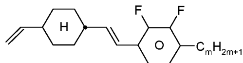
CVY-V-m
