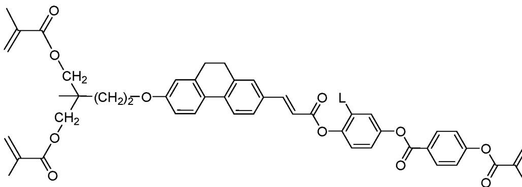
I-3-3a-5
