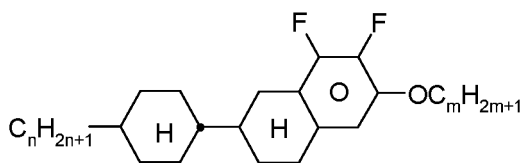
CTNap-n-Om
