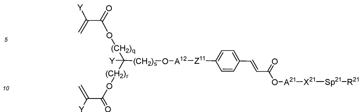
I-2-1
