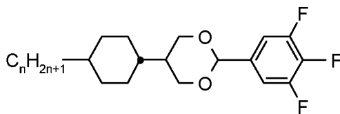
CDU-n-F
