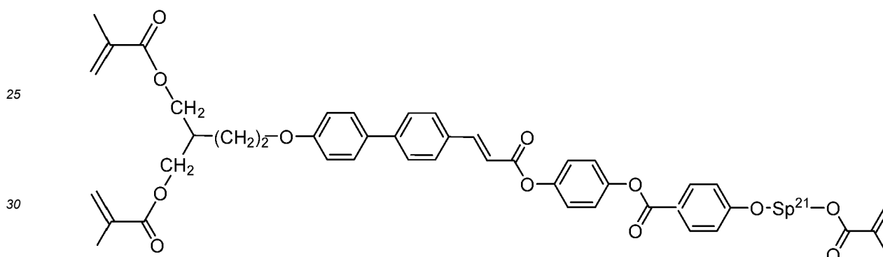
I-4-1a-1
