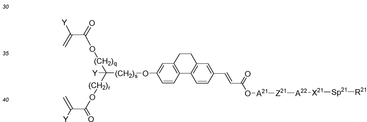
I-3-3
