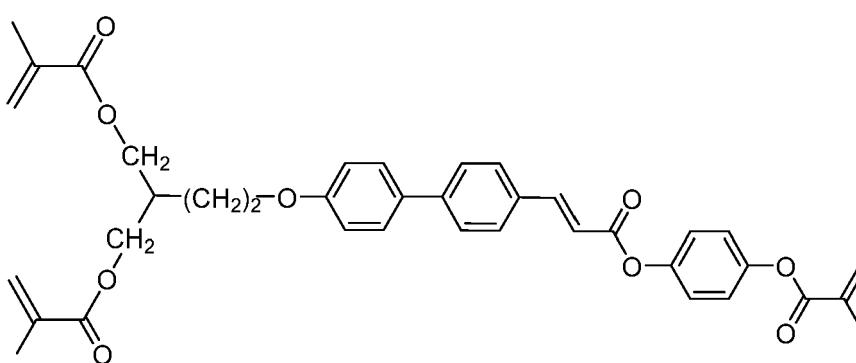
I-2-1a-2
