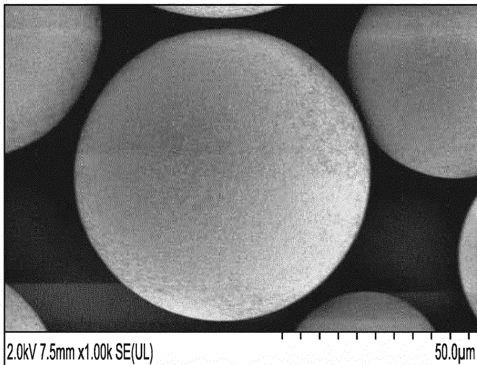
FIG. 16C
