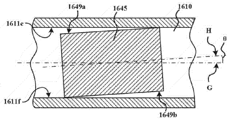
FIG. 18 (SECTION A-A)
