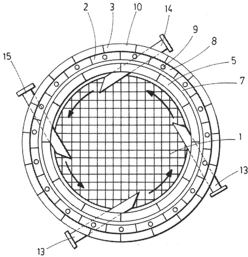
FIG.2 A-A'
