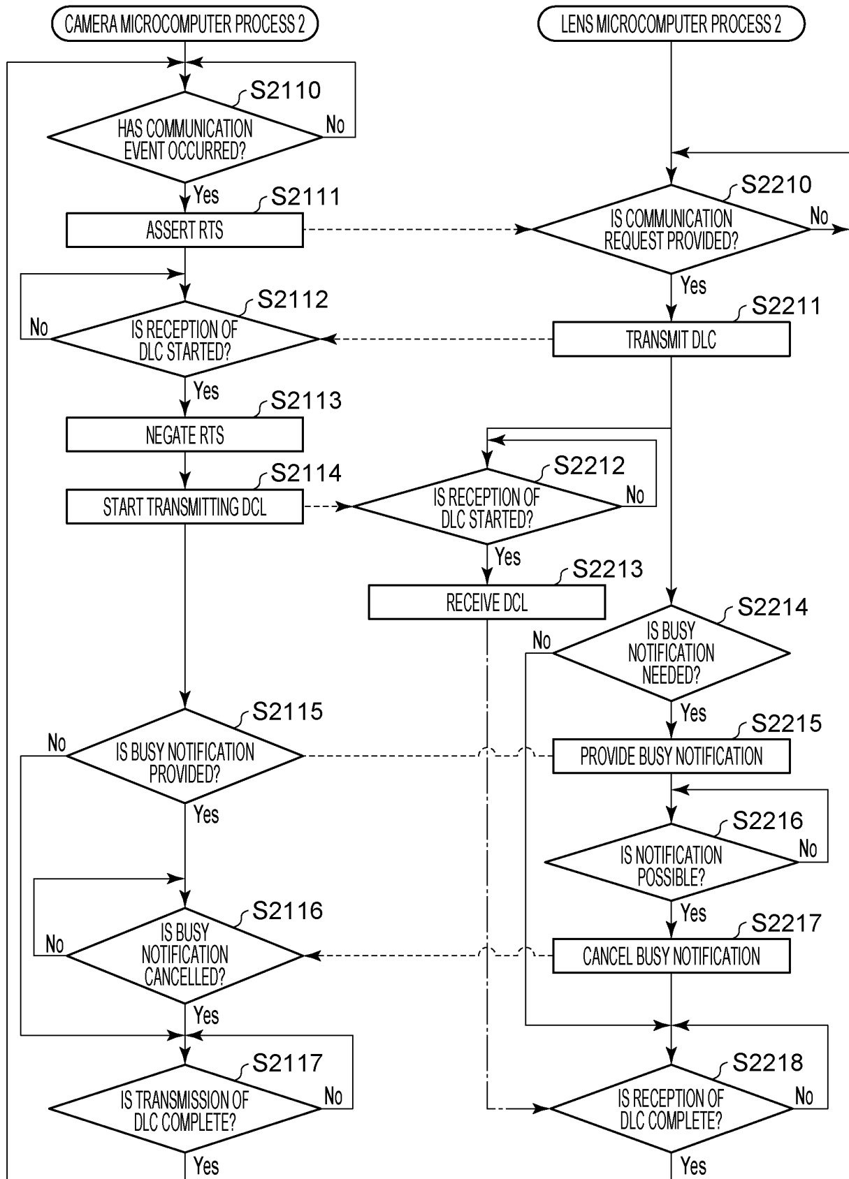
FIG. 23
