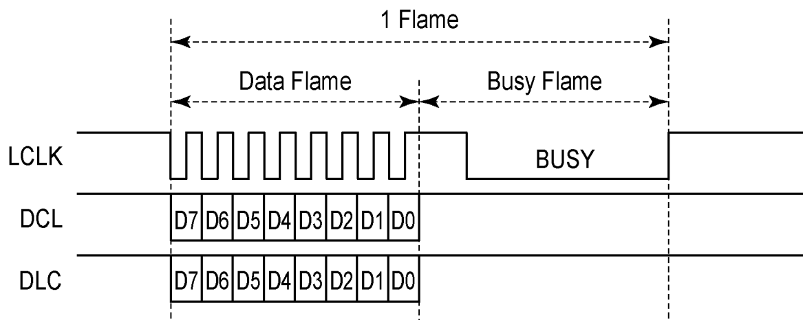
FIG. 19A
