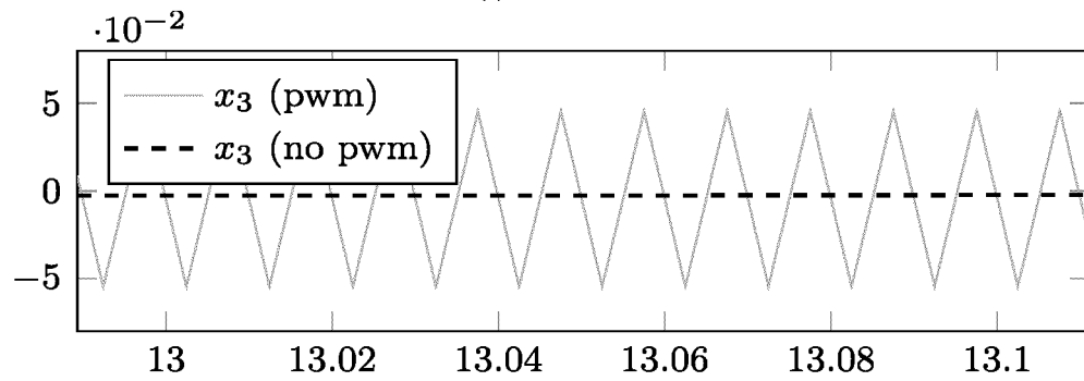
(d) State x_3 , zoom on (c).
