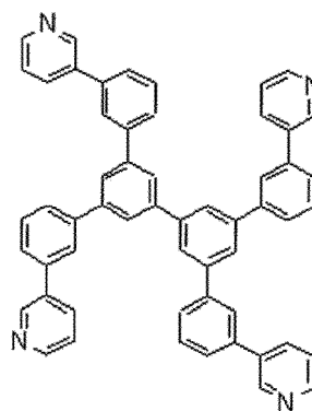
BP4mPy
