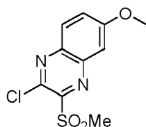
2-chloro-6-methoxy-3-(methylsulfonyl)quinoxaline
