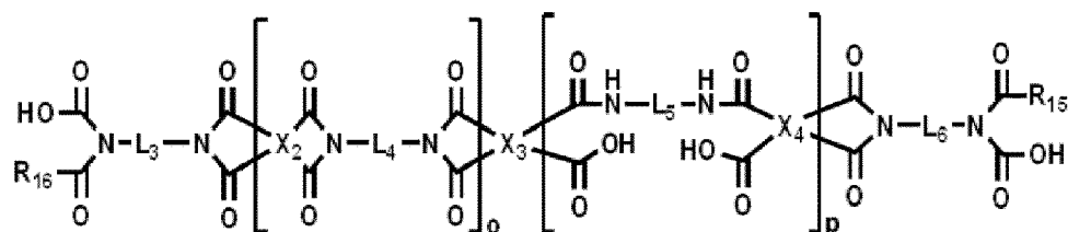
[Formula 5]
