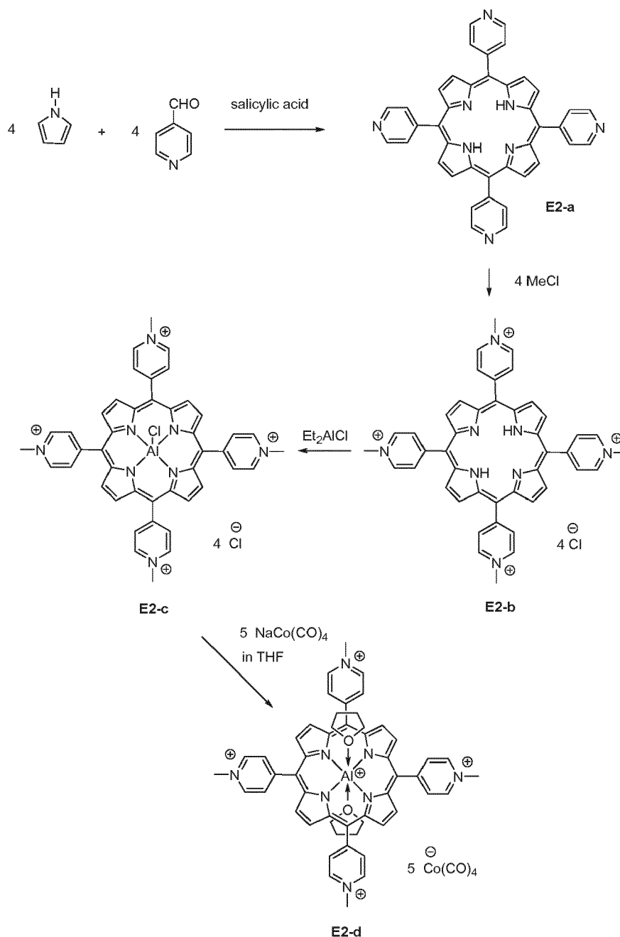
Scheme E2
