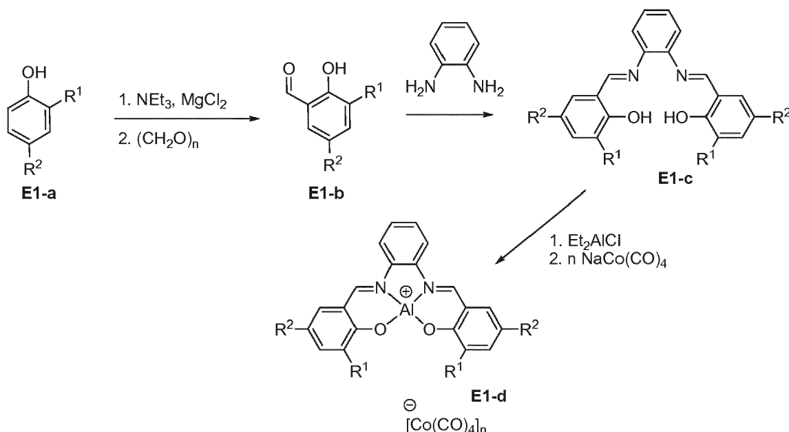
Scheme E1
