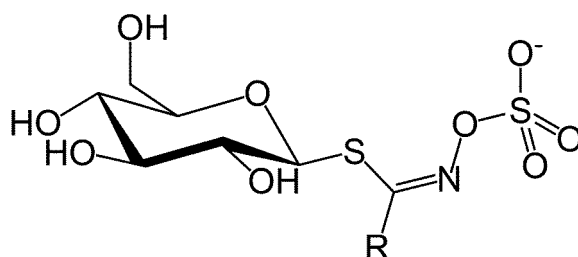
【Chemistry Figure 1】
