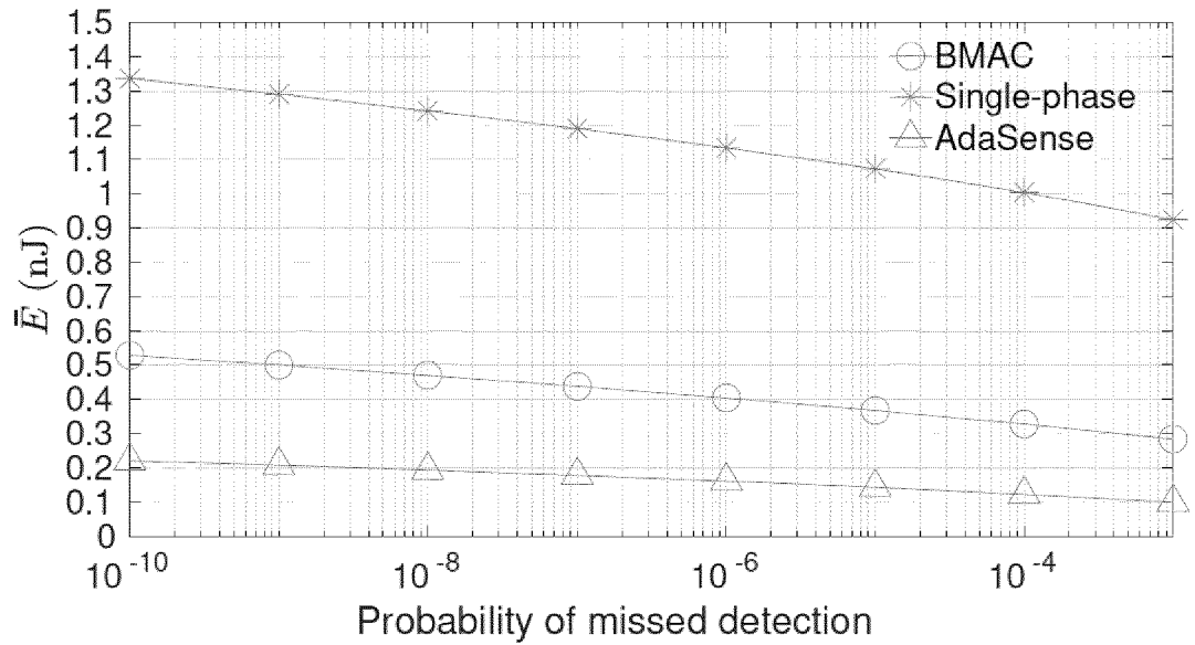
(d) n = 50 , P = -60\text{dBm} , P_{\text{FA}} = 10^{-5} . Energy savings 59%-65%.
