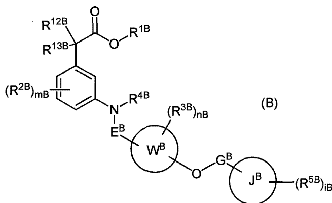
[Chemical 3]
