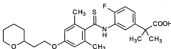
35 [Chemical 64]
