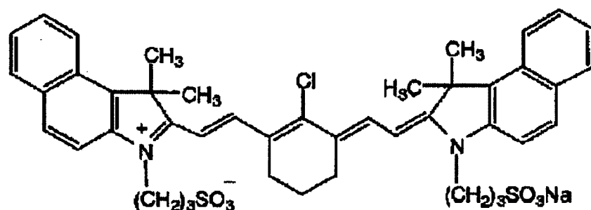
( IR-9 )
