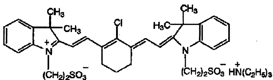
( IR-8 )
