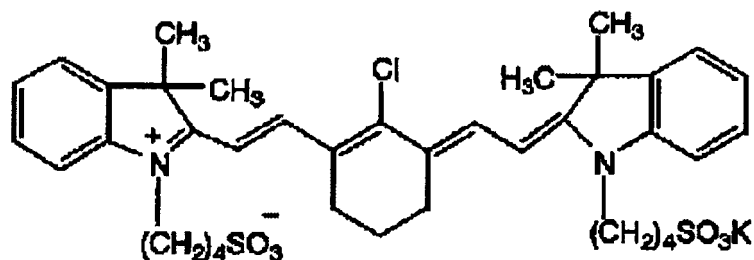
( IR-7 )
