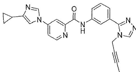
N-(3-(4-(but-2-ynyl)-4H-1,2,4-triazol-3-yl)phenyl)-4-(4-cyclopropyl-1H-imidazol-1-yl)picolinamide;
