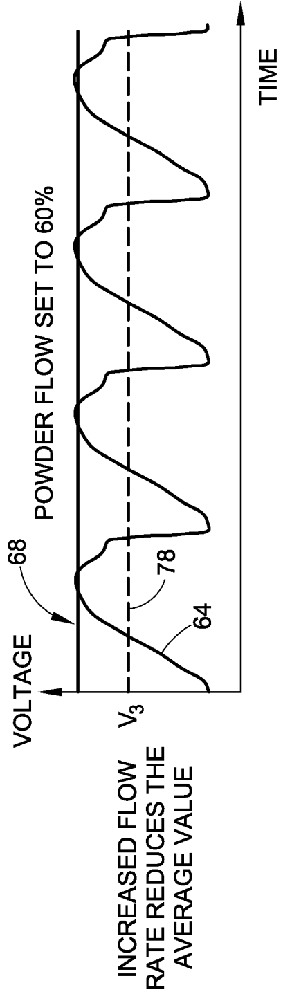
FIG. 4E
