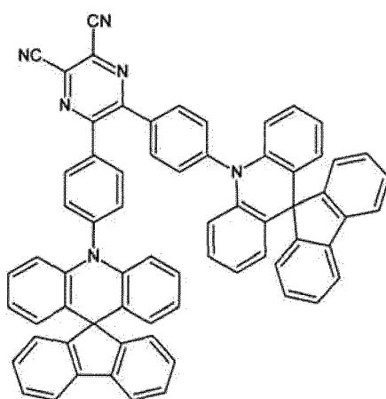
(I-8)
