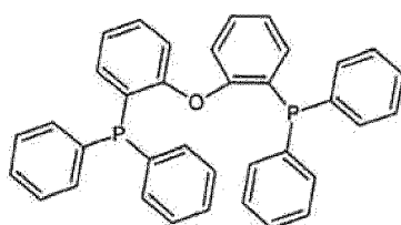
(e138)
