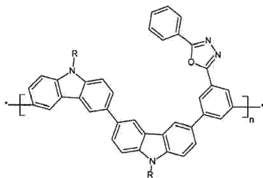
(e137)
