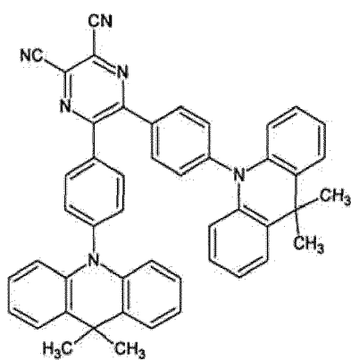
(I-9)
