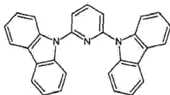
(e140)
