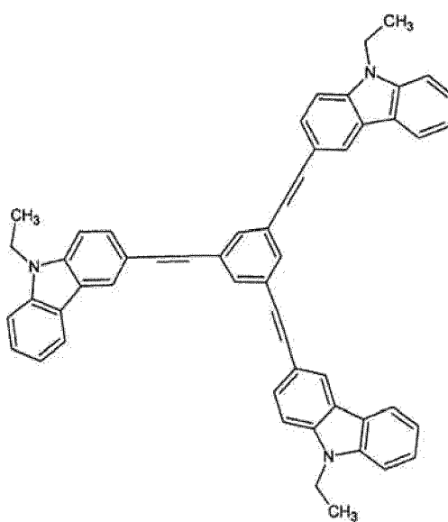
(ht18)
