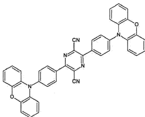
(II-4)
