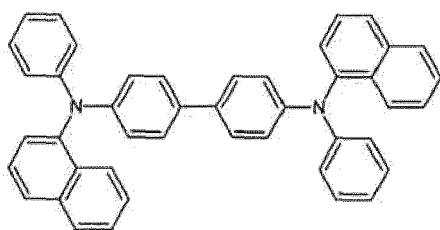
( \alpha -NPD)
