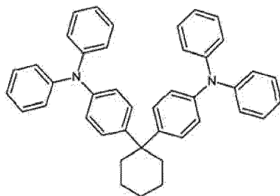
(TAPC)
