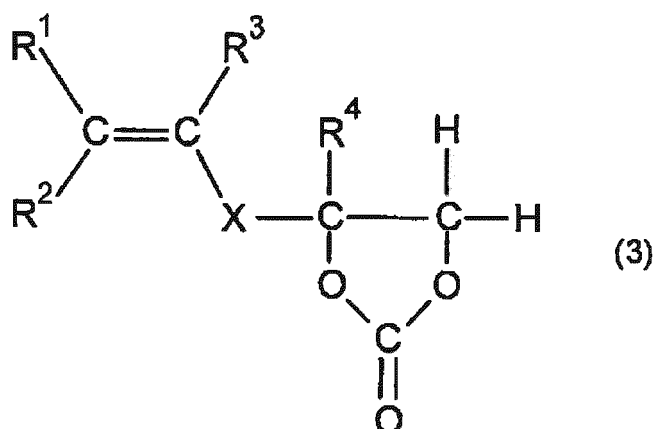
[Chem. 3]
