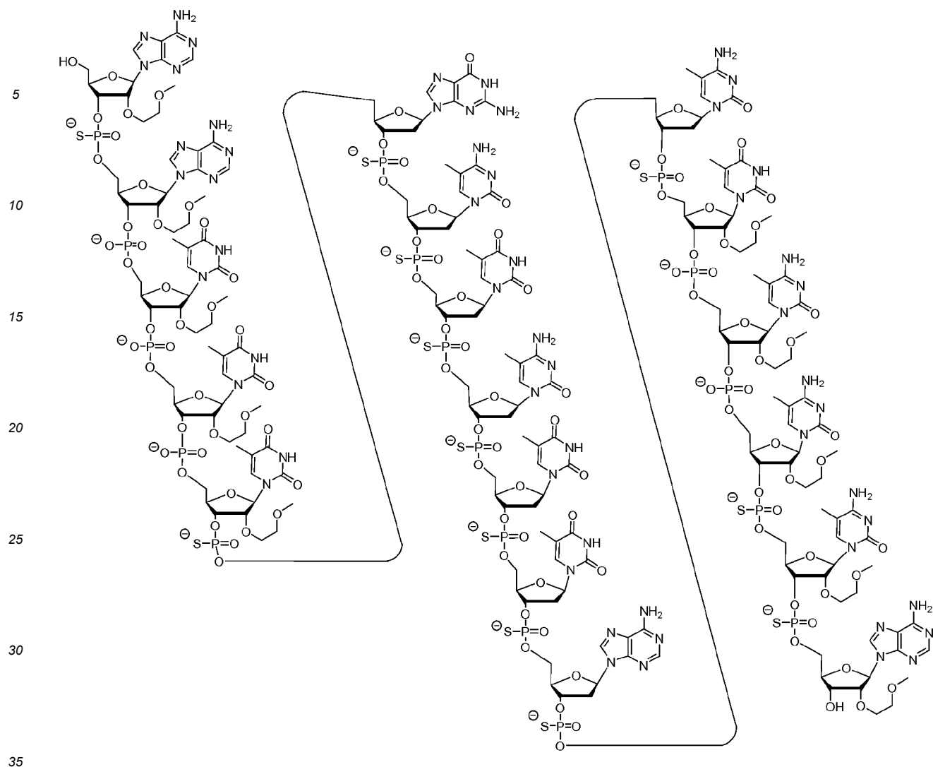
(Va)
