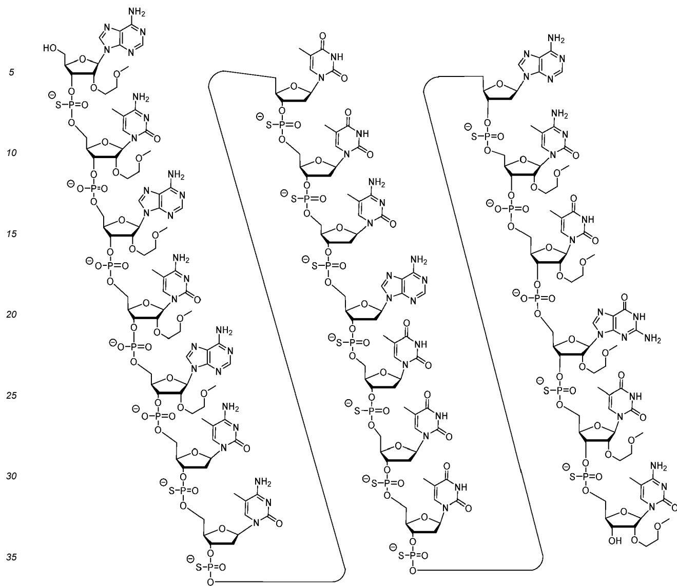
(IIa)
