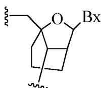
(J)
