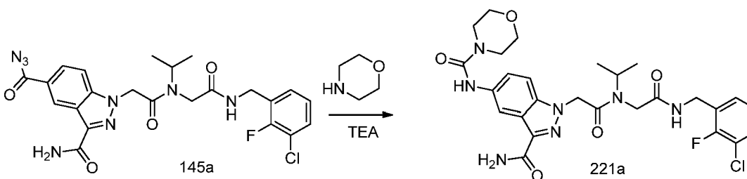
Scheme 221
