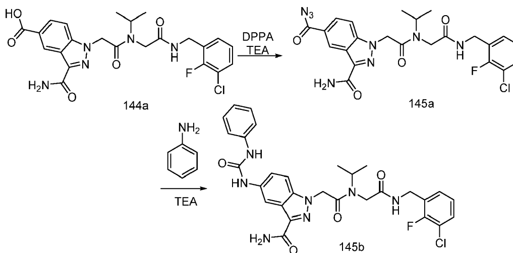
Scheme 145
