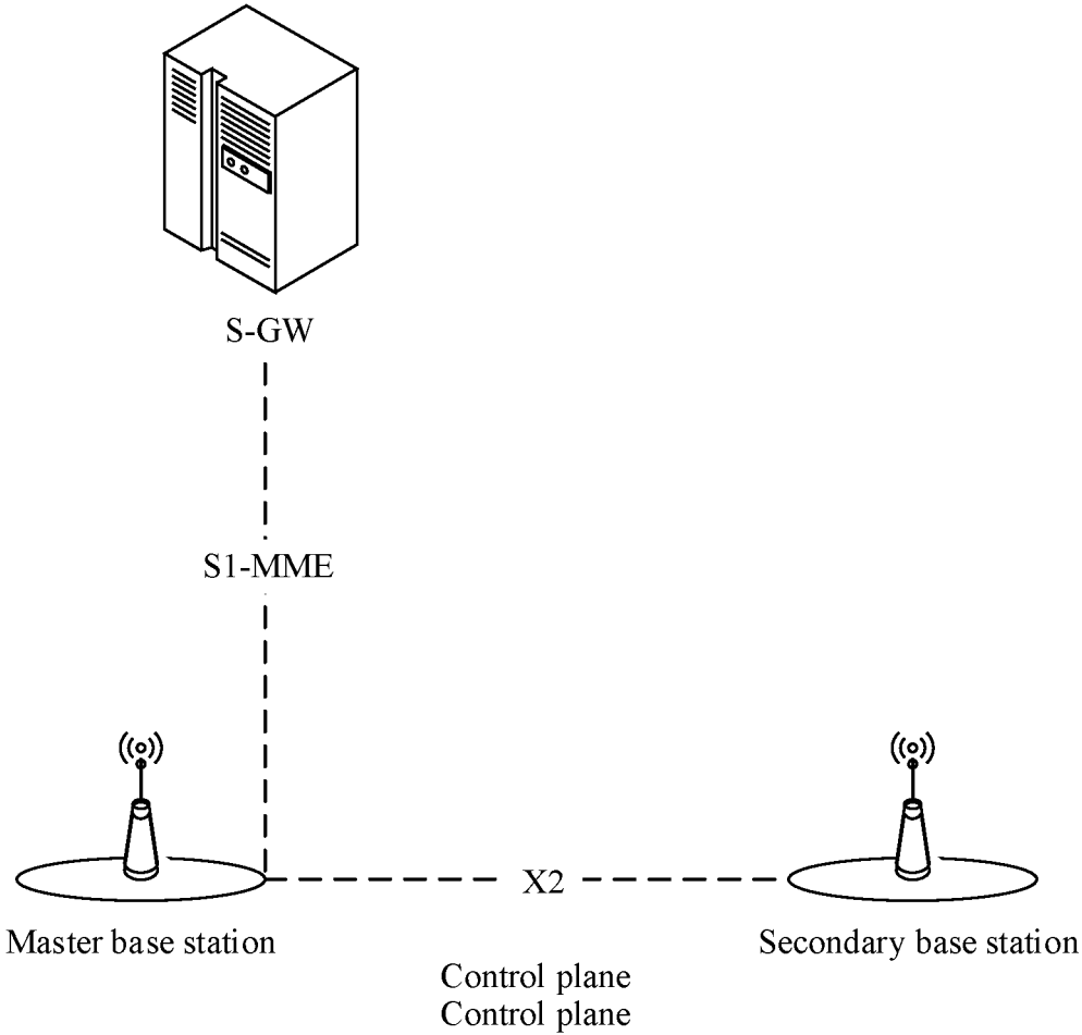
FIG. 1A
