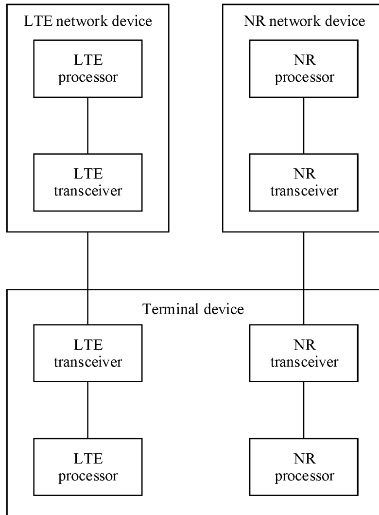
FIG. 6B
