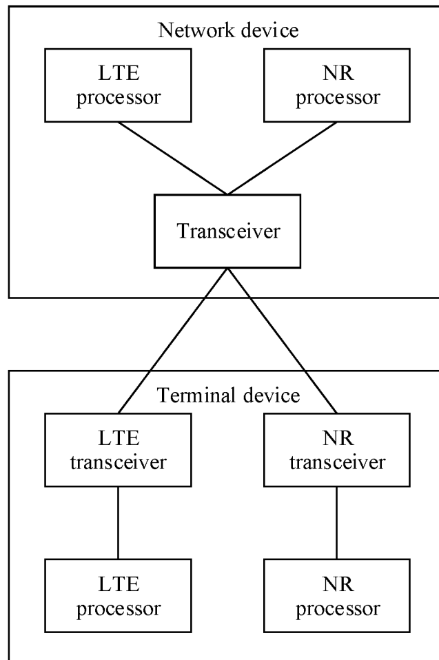
FIG. 4B
