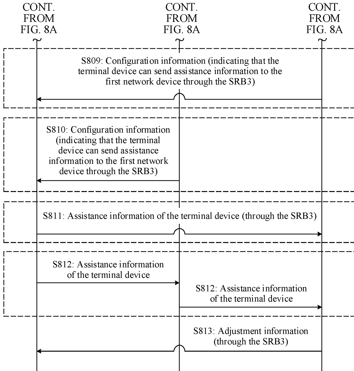
FIG. 8B
