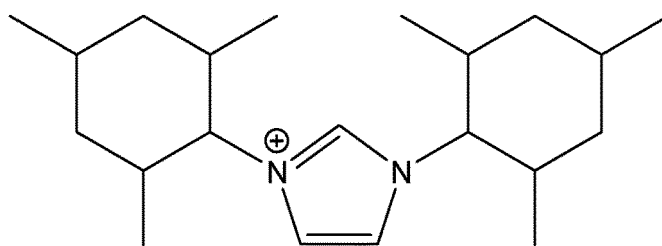
[Chem. 45]
