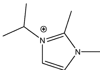
[Chem. 55]
