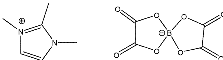
[Chem. 25]
