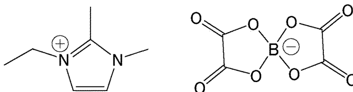
[Chem. 6]
