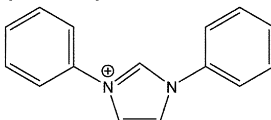
[Chem. 45]
