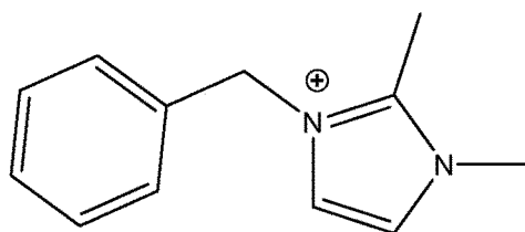
[Chem. 58]
