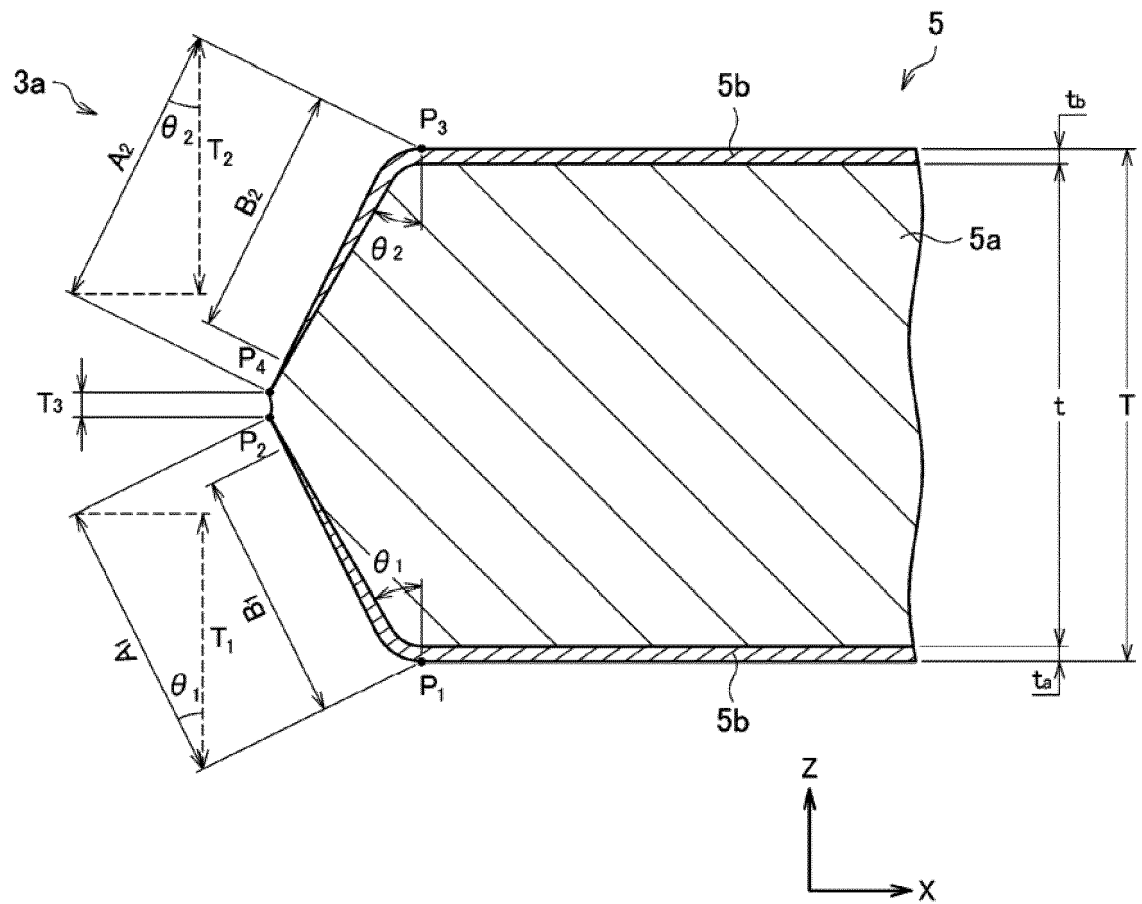
FIG. 23
