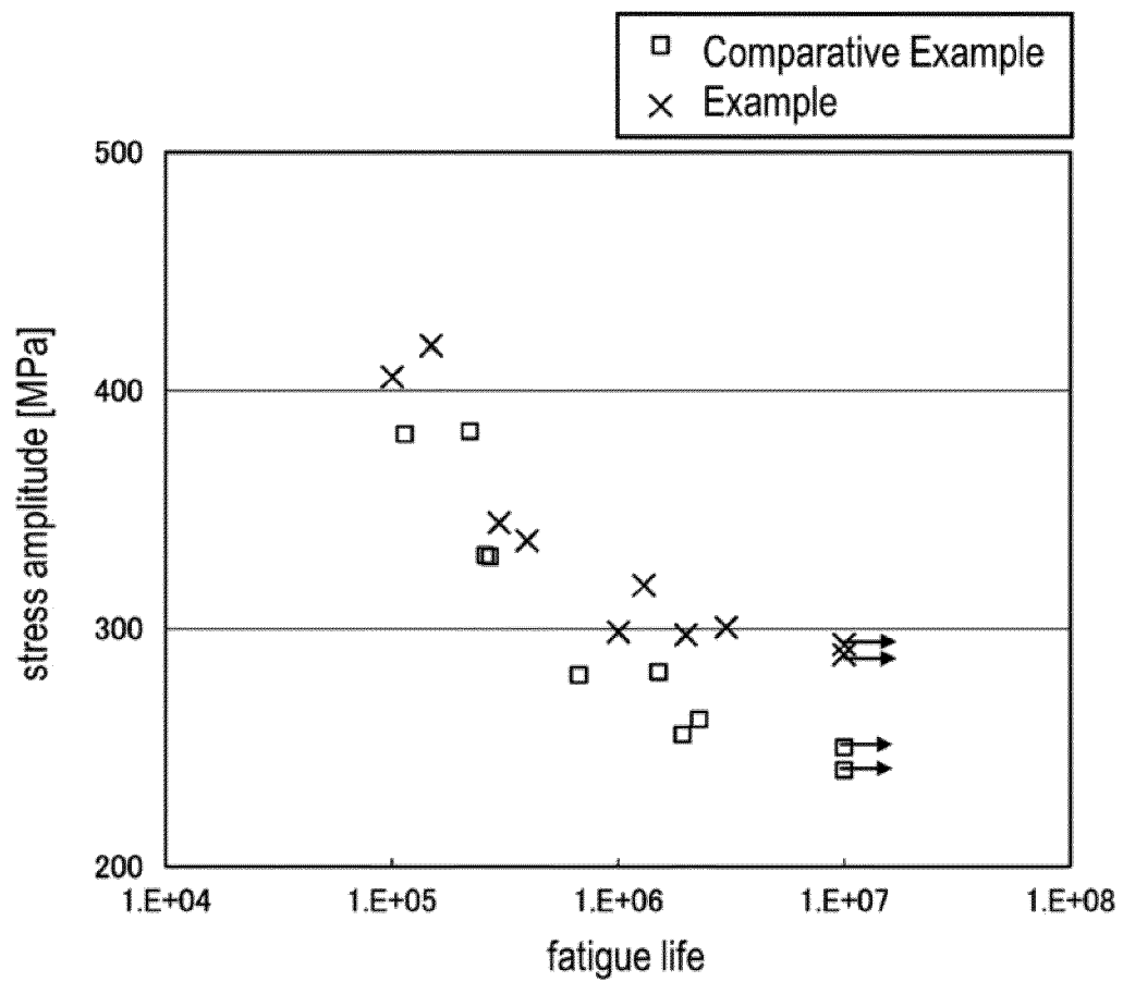
FIG. 34
