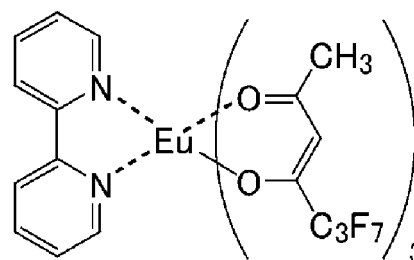
[Eu(FPD) 3 ]bpy
