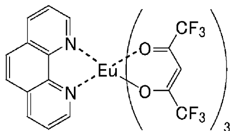
Eu(HFA) 3 phen
