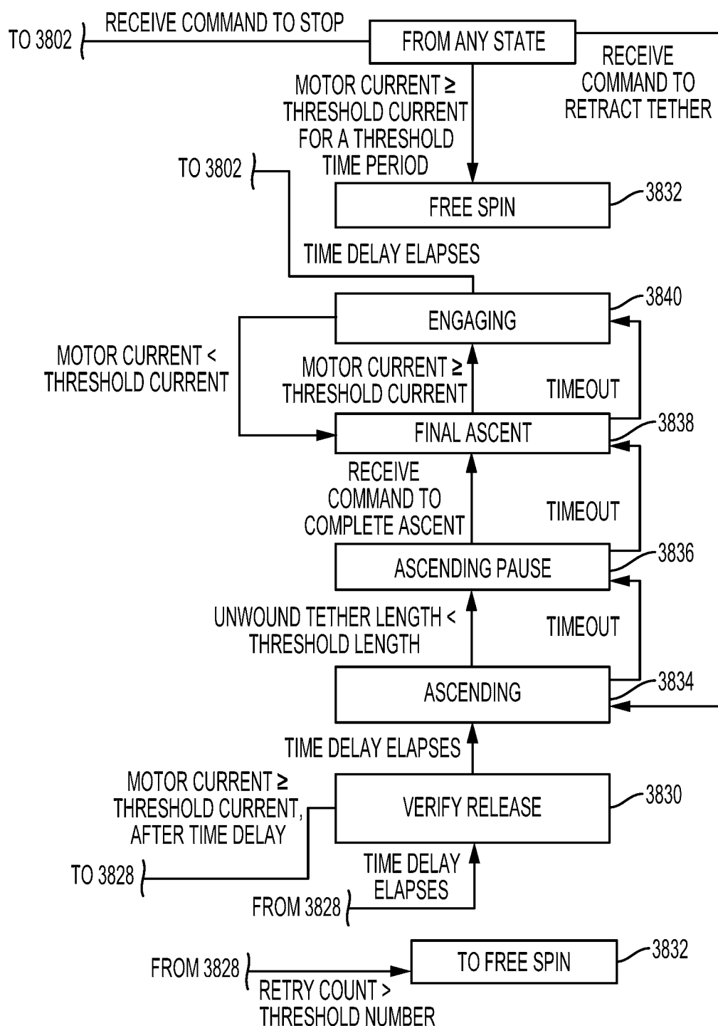
FIG. 38C
