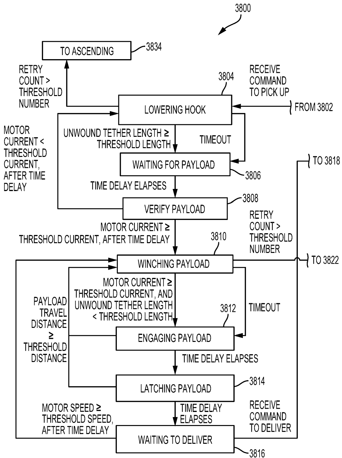
FIG. 38A
