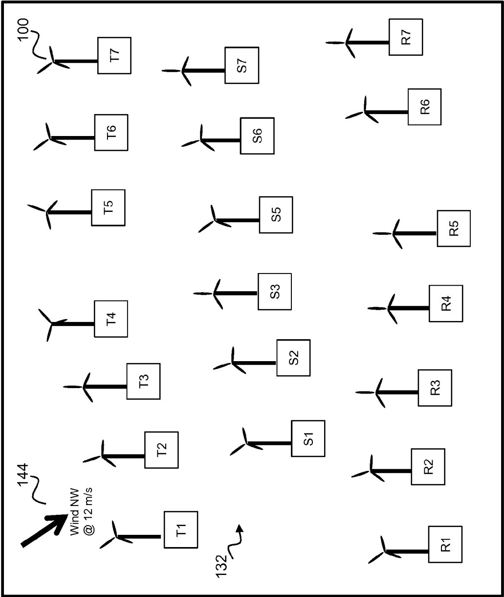
FIG. 10A
